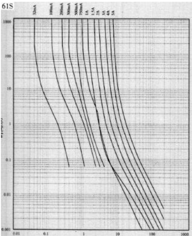
电流-时间曲线图
