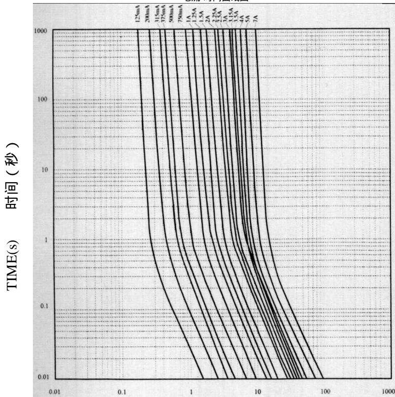
电流-时间曲线图
